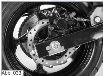
Hinterradbremse
