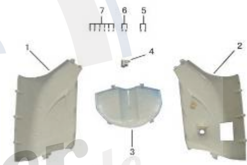
A6 - Verkleidungsteile ( Front bzw. Batterie)
